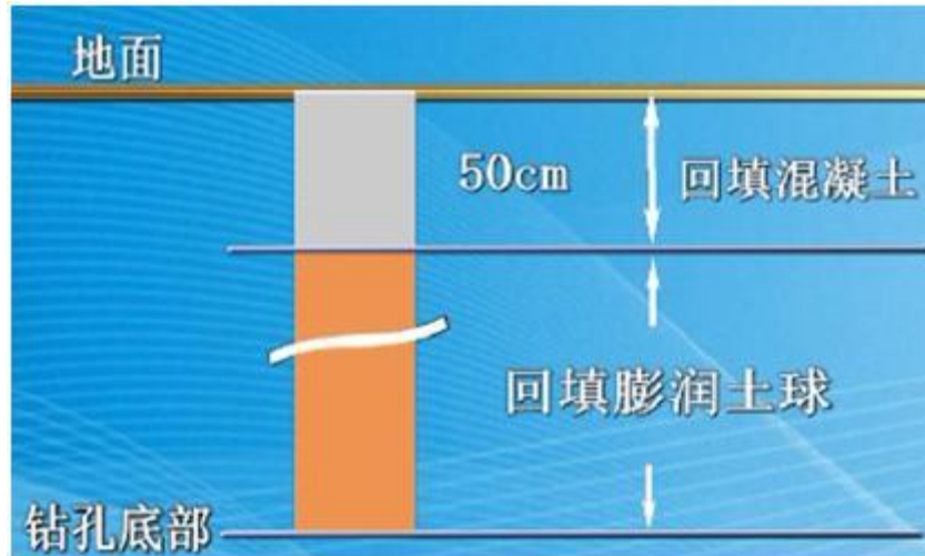
图 7.2-1 封孔要求
