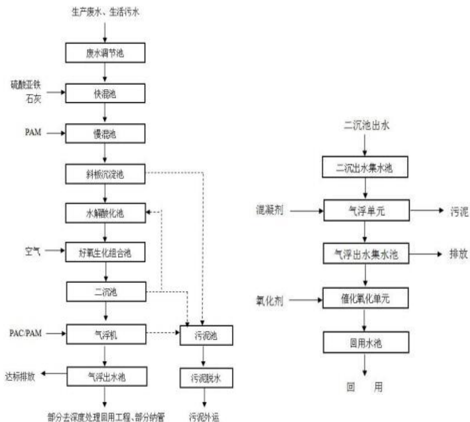
图 4.1-3 废水工艺流程图
