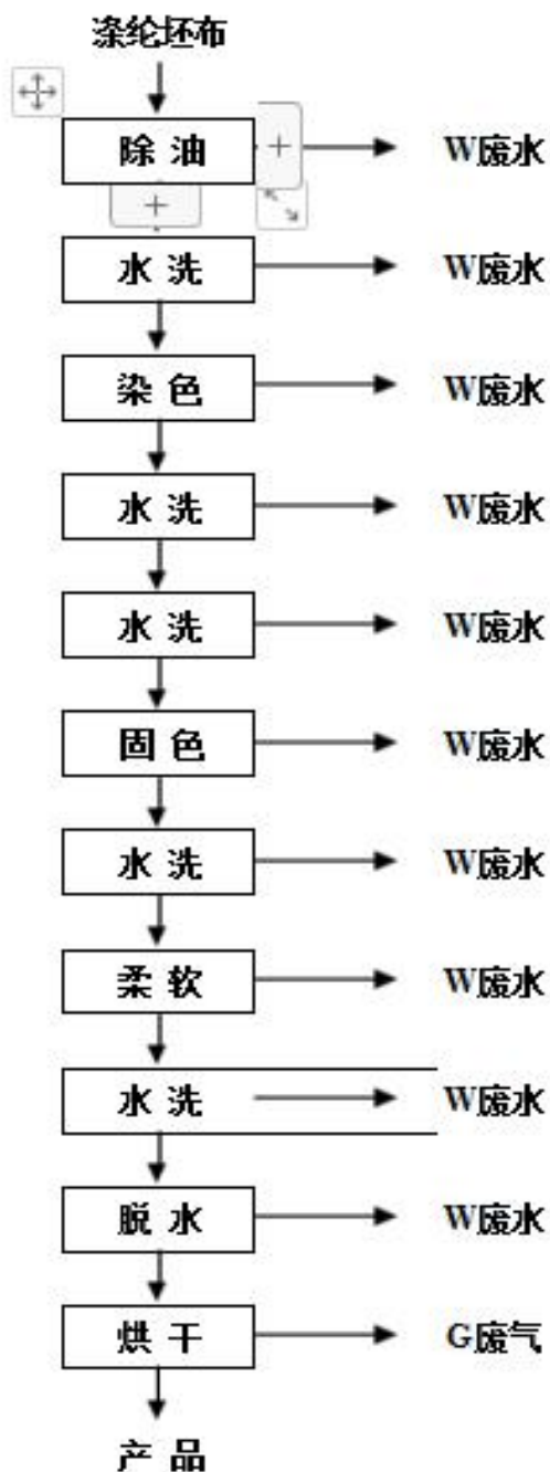
图4.1-1 染色加工生产工艺流程图
