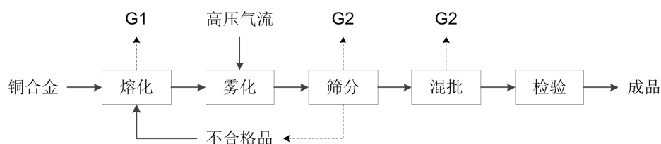
图4.1-3 整体生产工艺流程图
